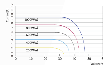
LNSF-335P/I-V
